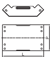
Поворот на 90° вертикальный внутренний
