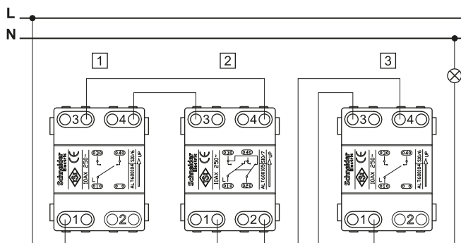
Управление одной нагрузкой с трёх мест с перекрестным переключателем
