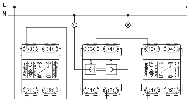
Управление двумя нагрузками с двух мест (2 переключателя + 1 двухклавишный переключатель)
