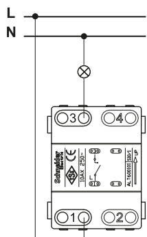
Одноклавишный выключатель
