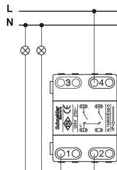
Двухклавишный выключатель
