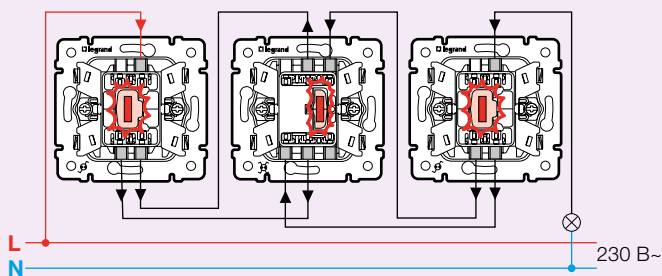
Переключатели на 2 направления и промежуточный переключатель с подсветкой (управление с 3-х мест) 7 743 26 + 7 743 48 + 7 743 26 (или 7 744 26 + 7 744 48 + 7 744 26)
