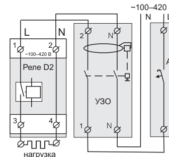
Схема 1. Подключение автоматического выключателя и УЗО с транзитом нуля через реле
